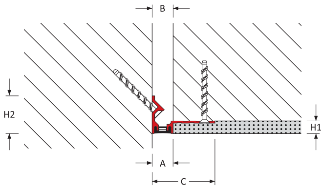
MaxAtec 130 : A09
